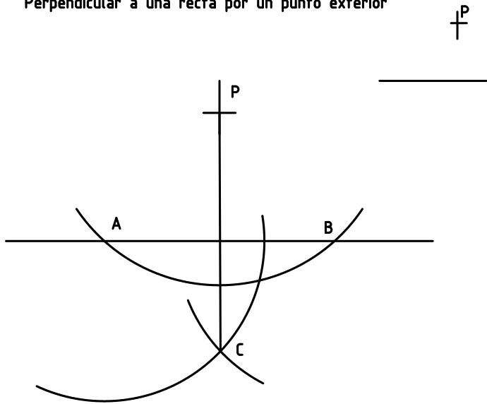
Perpendicular a una recta por un punto exterior
