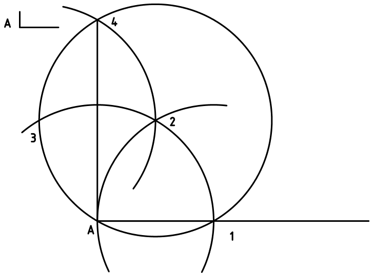
Perpendicular a una semirecta en su extremo A
