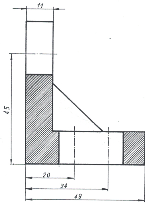
SECCIÓN A-B
