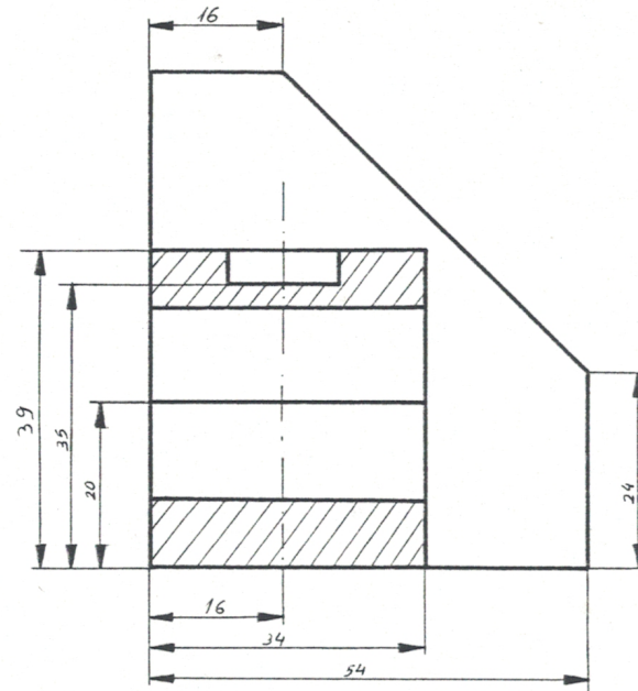
Sección AB
